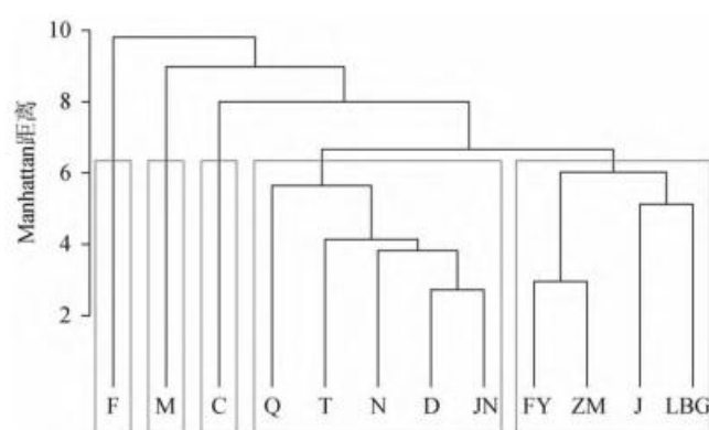
图3 基于香气电子鼻分析结果不同香型白酒的聚类分析
