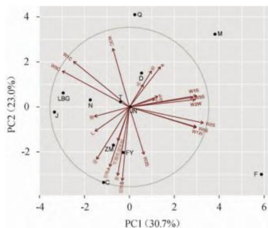
图4 不同香型白酒主成分分析结果
